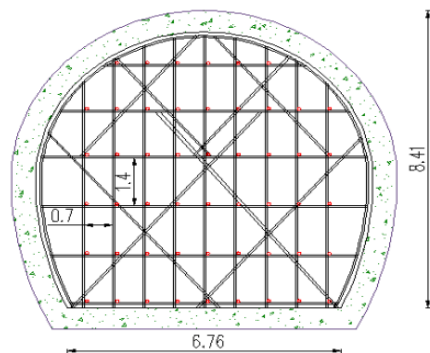
图1 是本支架衬砌结构示意图
